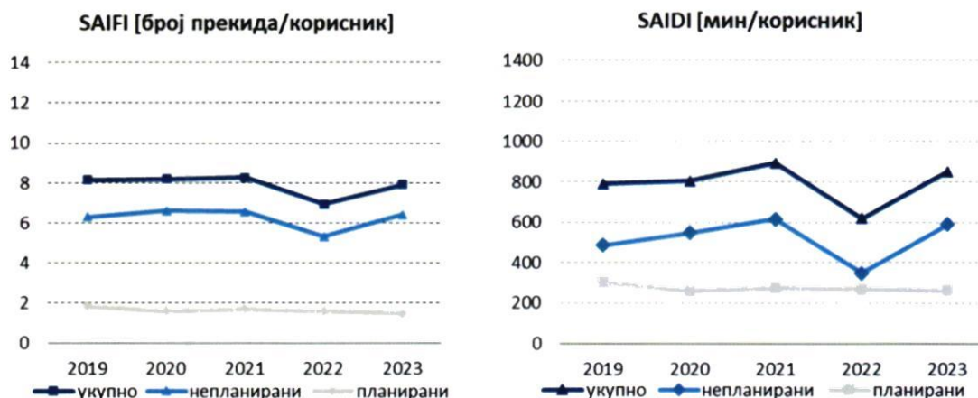
Слика 3-19: SAIFI и SAIDI за период 2019 - 2023. година
