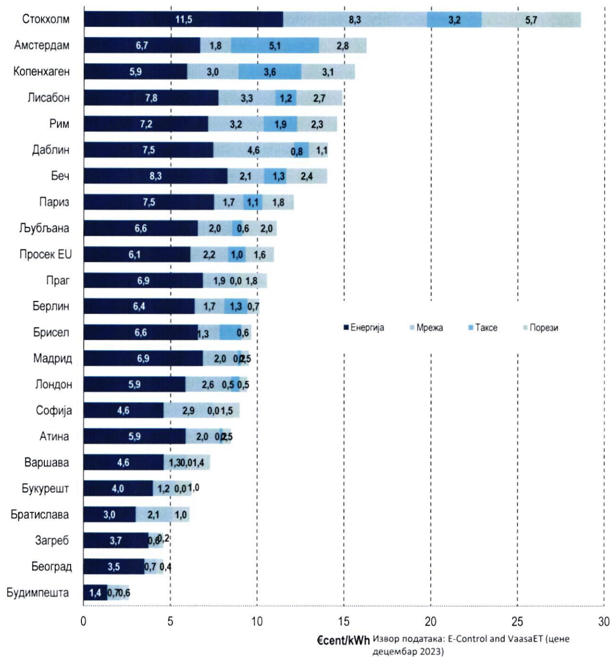
Слика 4-9: Структура цене природног гаса за домаћинства у појединим европским главним градовима у децембру 2023. године
